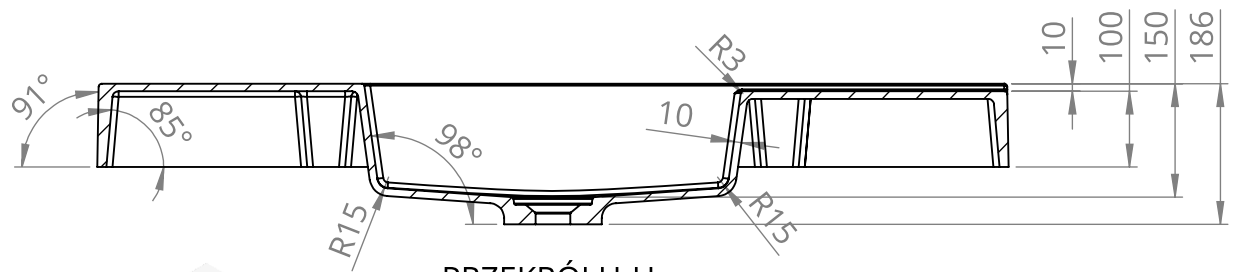
PRZEKRÓJ H-H SKALA 1 : 10
