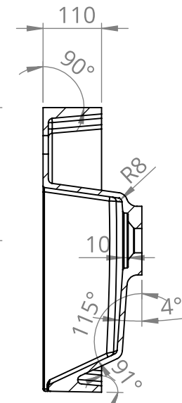
PRZEKRÓJ K-K SKALA 1 : 10
